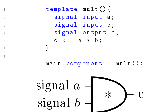
Ejemplo 1.2: Ilustración comparativa código-circuito
